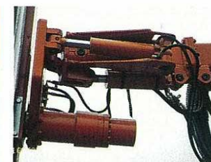
旋回装置
